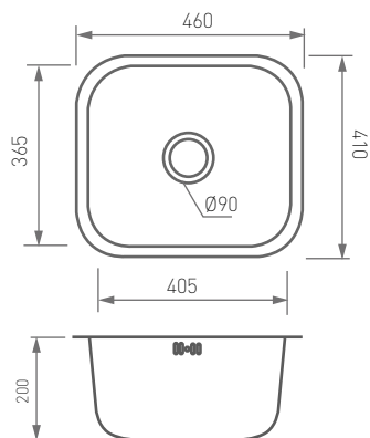
Vistas acotadas
